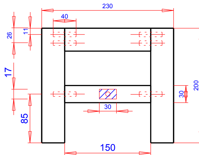
- Seitenansicht -
