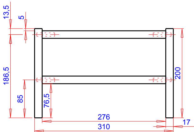
- Vorderansicht -
