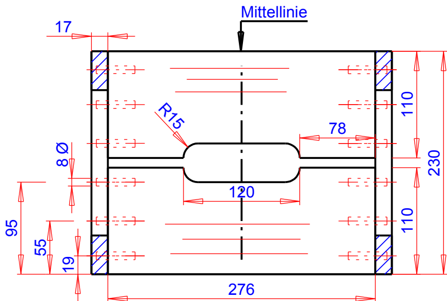
- Draufsicht -
