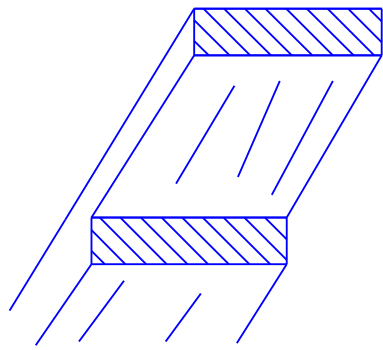
Perspektivische Darstellung der Ecküberblattung
