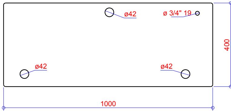
Draufsicht
